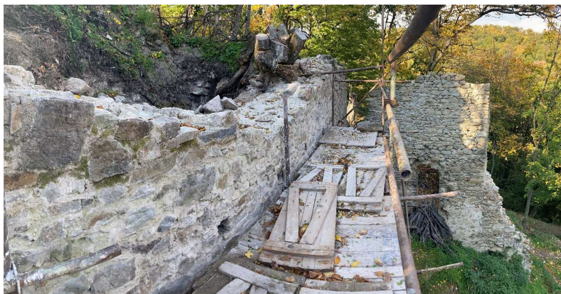
Obr. Sanačný zásah M5/2022: Oprava hornej časti severného úseku východnej hradby
